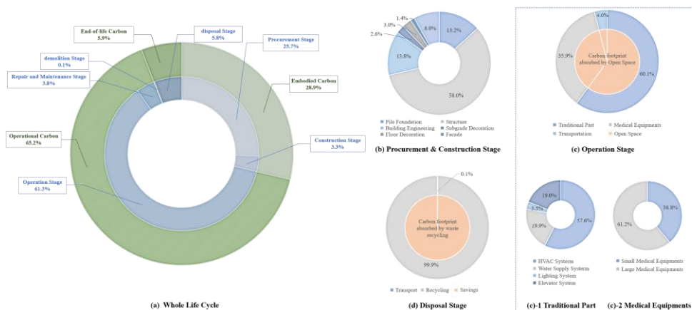
图 3-8 虚实数据融合医院全生命周期碳排放预测方法计算结果
