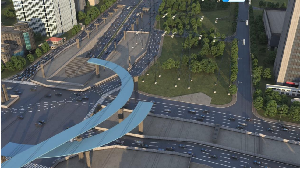
图 3-5 受限空间下吊装方案仿真模拟
