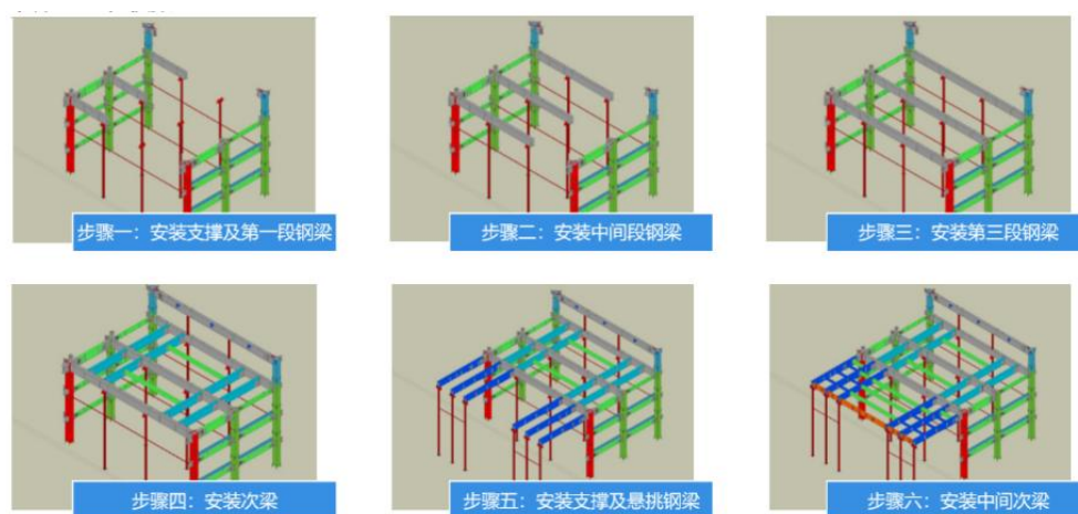
图 3-15 大跨度悬挑梁安装步骤模拟
