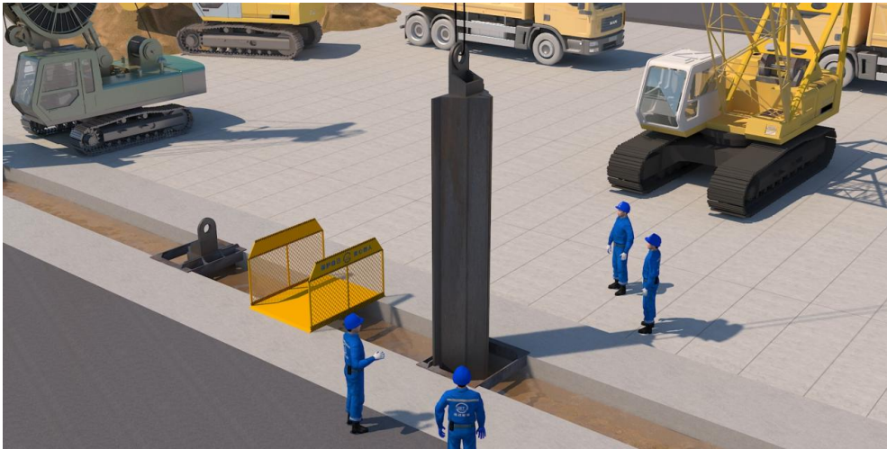
图 3-8 地下连续墙施工专项方案可视化技术交底
