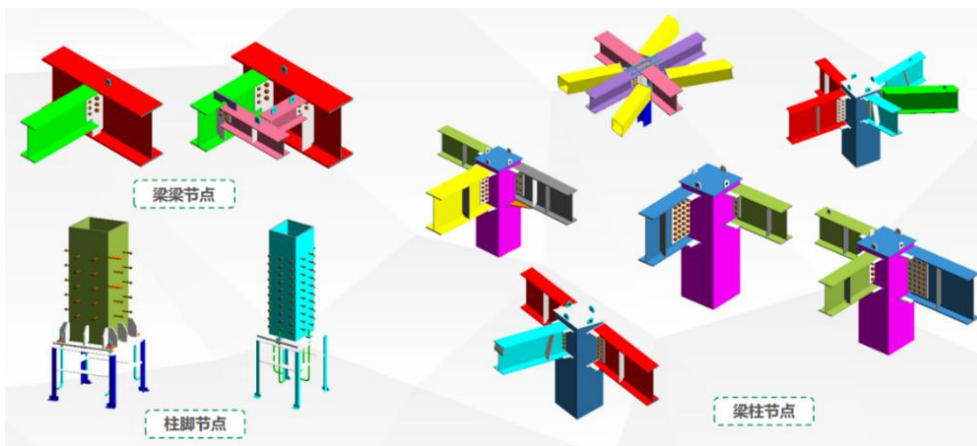
图 3-20 BIM 钢结构深化
