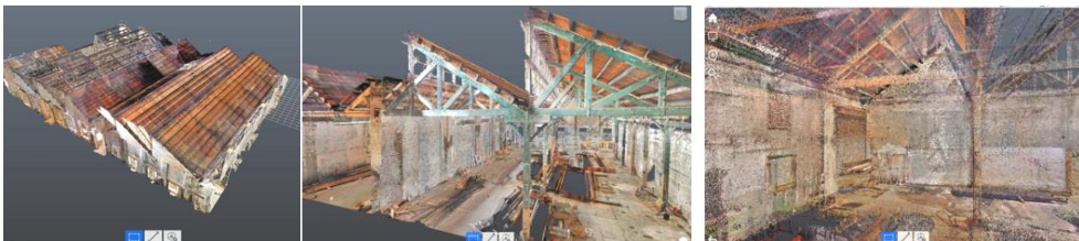
图 3-3 项目点云模型示意图
