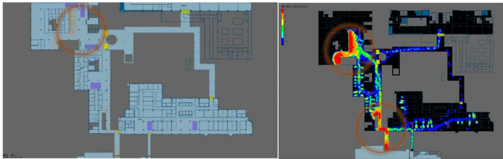
图 3-13 2F 一站式服务中心人群仿真模拟动态模型及最大密度图（优化前）
