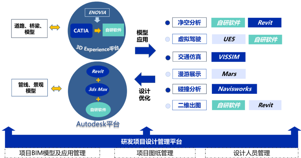
图 2-3 软件架构图
