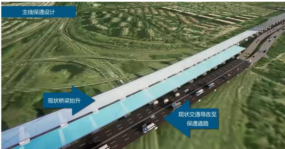
图 3-10 保通方案设计
