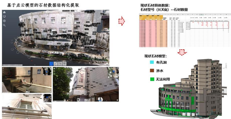
图 3-1 基于点云模型的石材数据结构化提取
