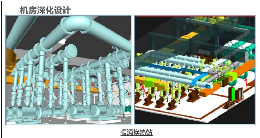
图 3-6 暖通换热站
