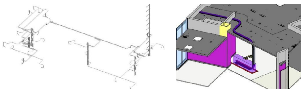
图 3-3 轨道物流系统模拟
