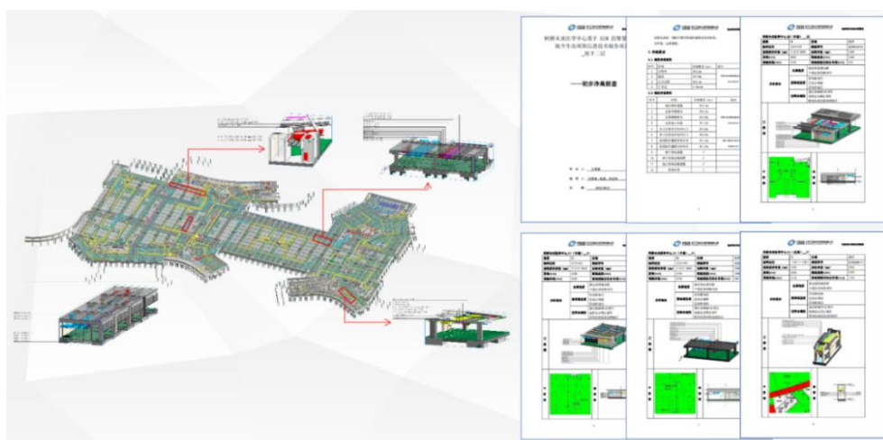
图 3-13 管线综合及净高分析
