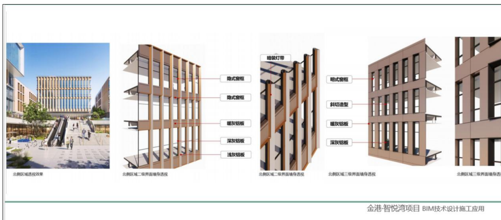
图 3-2 窗墙系统
