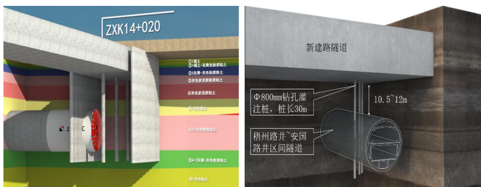
图 3-10 盾构掘进前拔桩方案制定
