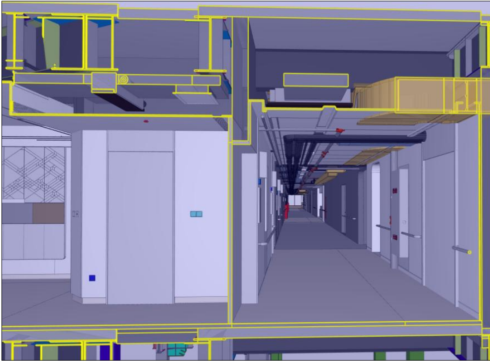
图 3-11 装饰设计碰撞解决
