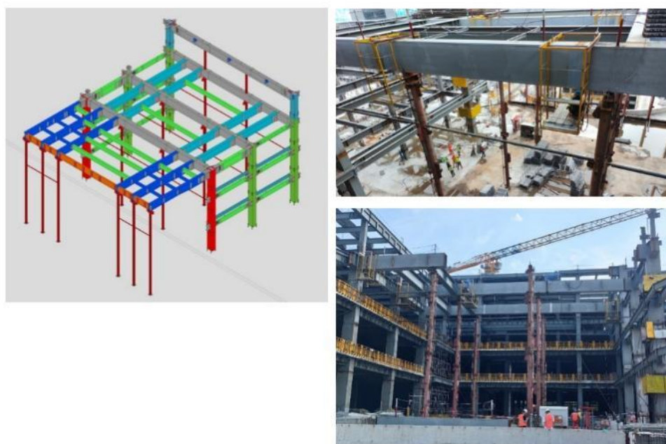
图 3-16 大跨度悬挑梁模拟与安装
