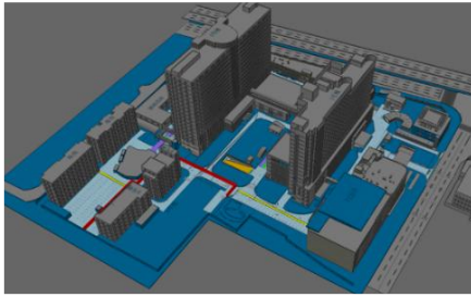
图 3-10 院区建筑场地 BIM 模型
