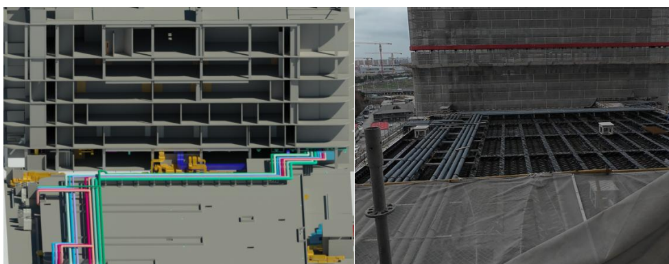
图 3-18 大管径主管模拟与安装
