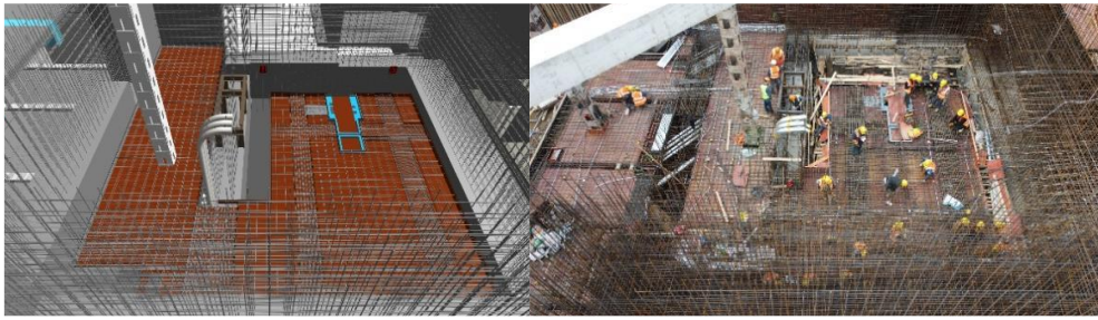
图 3-21 管线精准预埋技术
