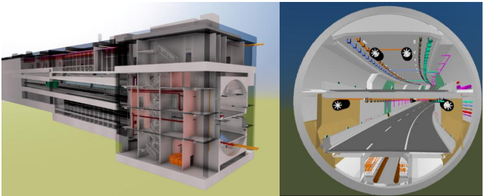
图 3-6 工作井及盾构段各专业集成
