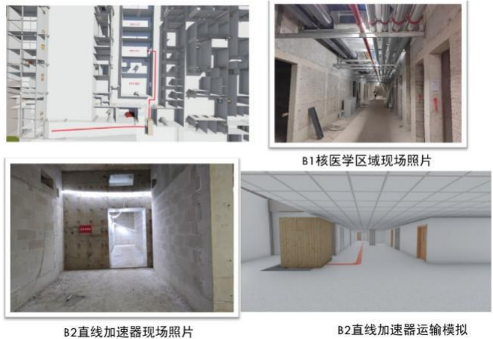
图 3-6 核医学科设备运输路线模拟
