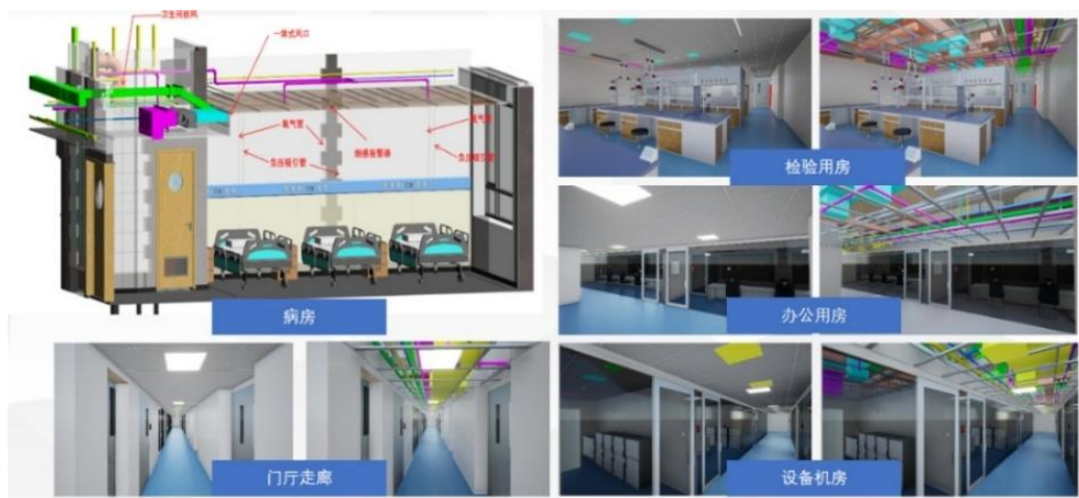
图 3-8 模块单元深化
