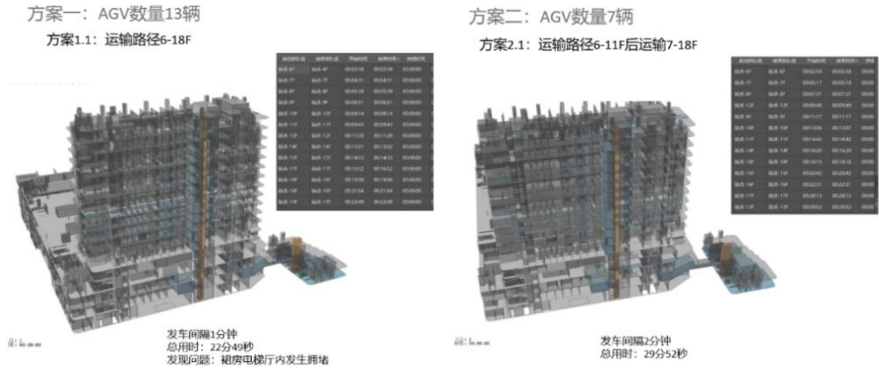
图 3-5 AGV 小车模拟界面及结果数据
