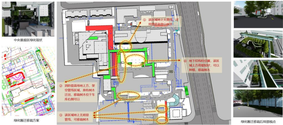
图 3-2 场地摸排及绿化搬迁模拟分析
