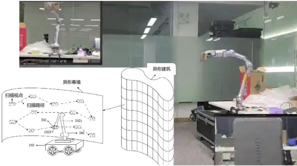
图 3-5 机械臂交互式自主观测系统
