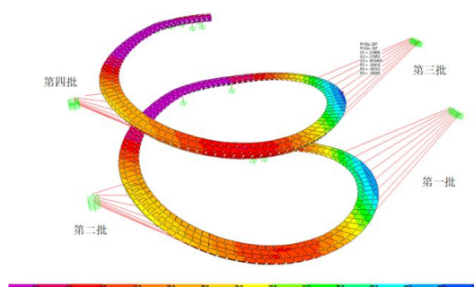
图 3-3 拉索张拉顺序
