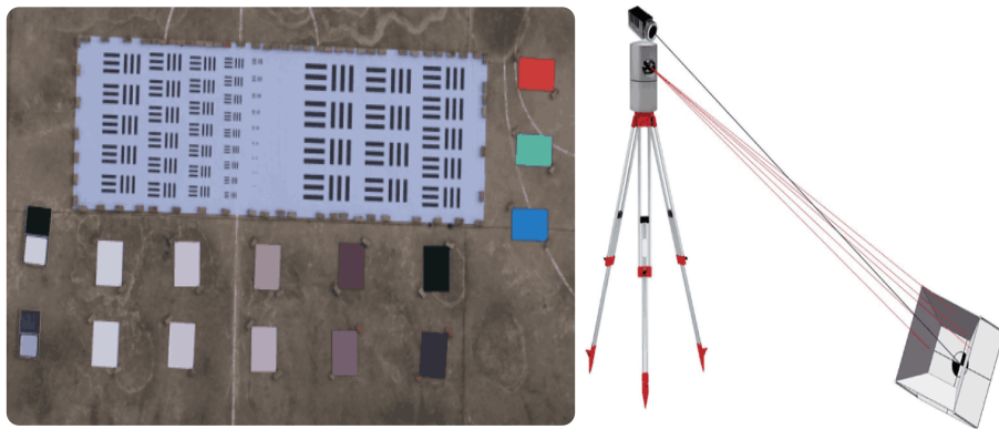
图 3-2 一致性检校装置
