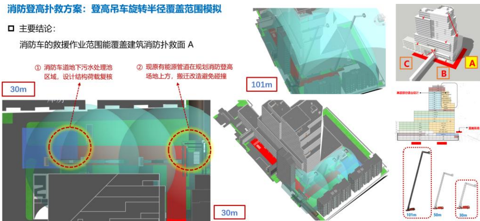
图 3-3 项目主要消防登高扑救场地及不同类型消防登高吊车模拟
