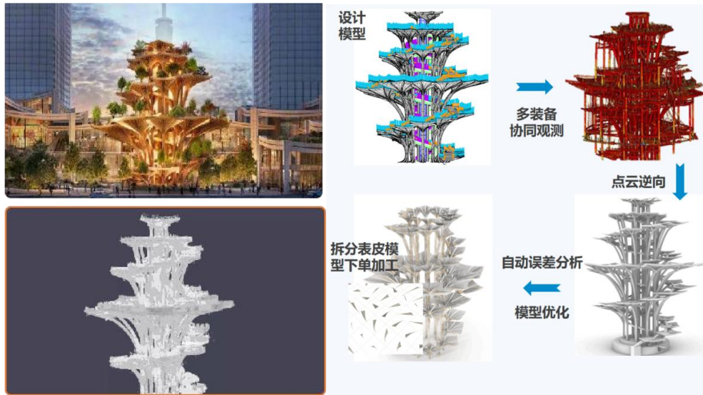
图 4-6 生命之树多装备观测点云逆向 BIM 模型
