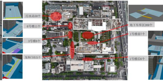
图 3-11 院内现有停车位分布模型（372 个）
