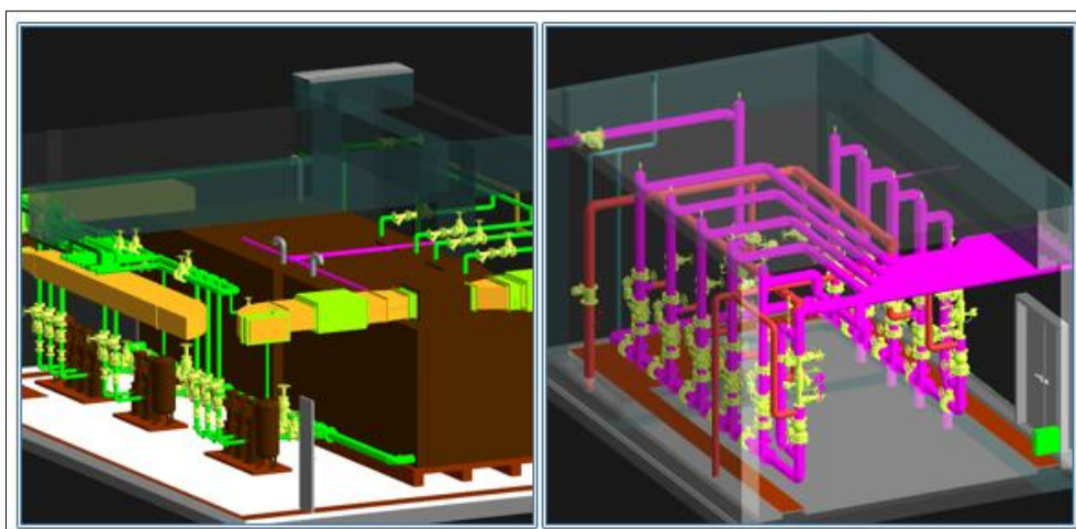
图 3-7 生活水泵房
